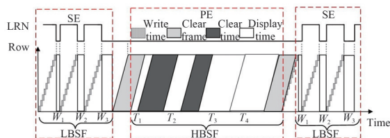
图4 DMFS原理图
