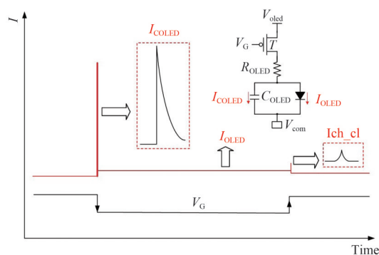
图3 OLED电流仿真图
