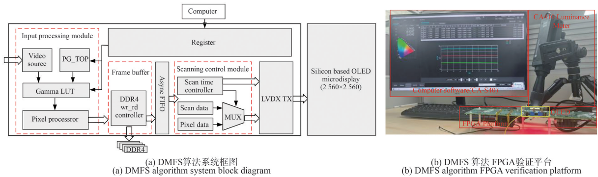
图 7 DMFS 算法电路原理图 Fig. 7 Schematic diagram of DMFS algorithm
