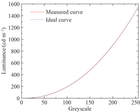
图 10 实测与理想 gamma2.2 灰阶曲线
