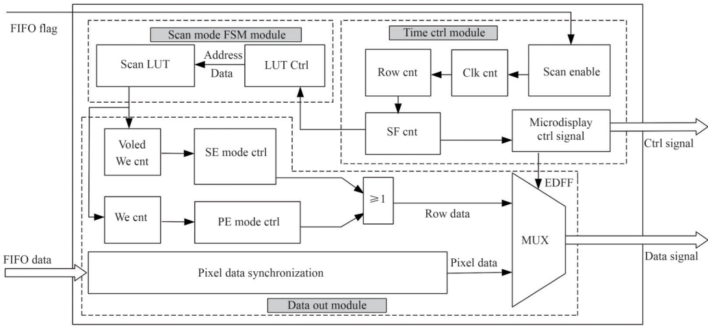
图 6 DMFS 扫描控制模块 Fig. 6 Scanning control module of the DMFS algorithm
